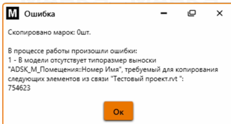
Рисунок 9 - Конфликт марок №3
