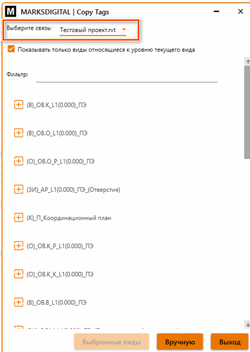
Рисунок 4 - Выбор связи
