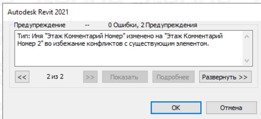
Рисунок 8 - Конфликт марок №2
