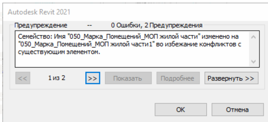
Рисунок 7 - Конфликт марок №1
